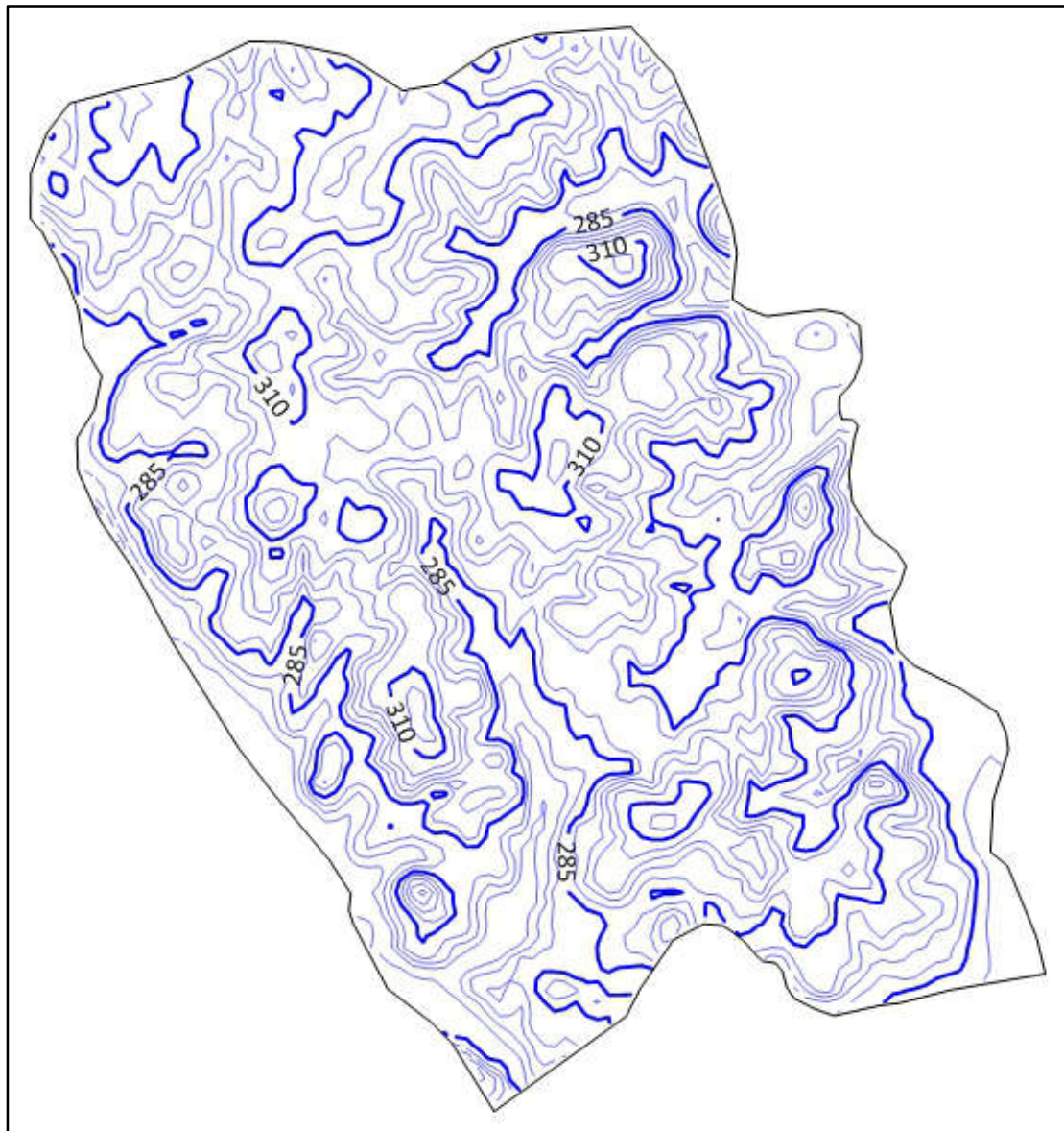
图 5.2.2-5 初始水位等值线图（2021.8）
