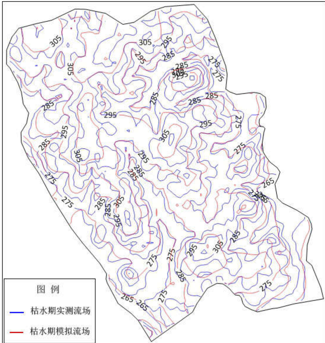
图 5.2.2-6 模拟区枯水期实测等水位线与计算等水位线对比图 (2021.11)
