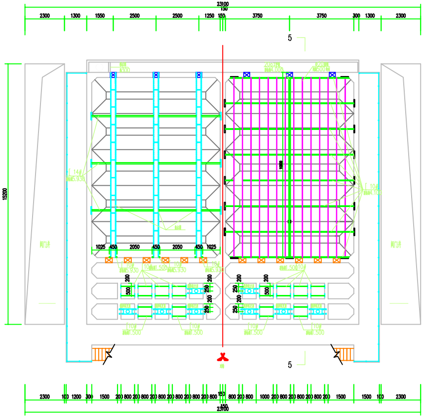
混凝沉淀池支架平面布置图
