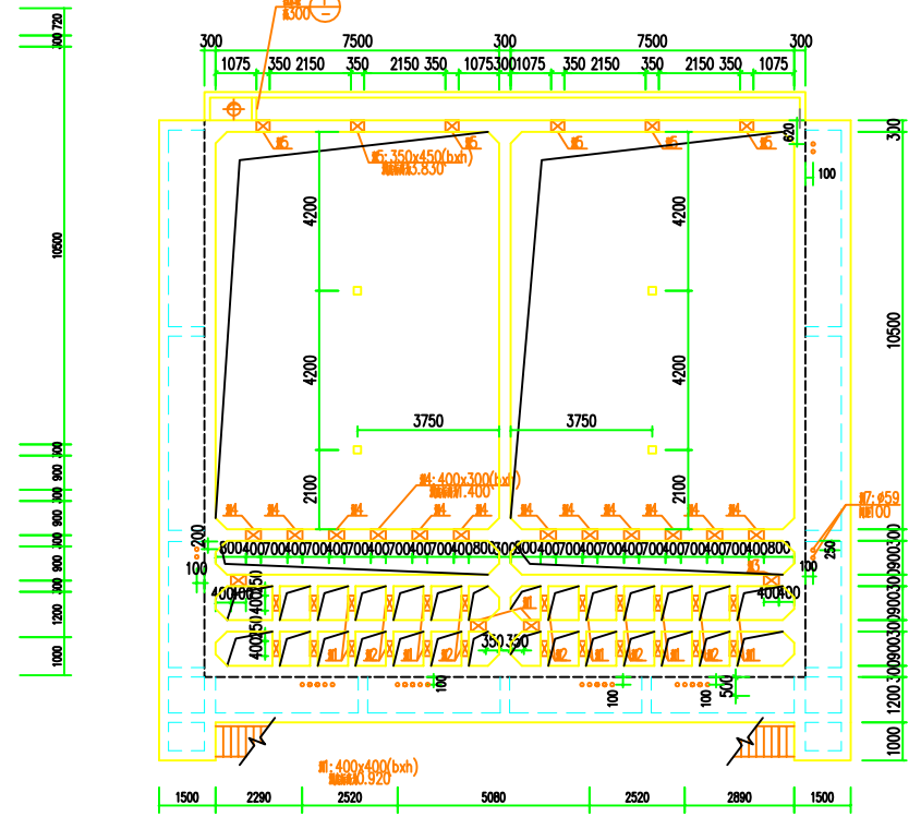
混凝沉淀池池壁及池顶板留洞布置图
